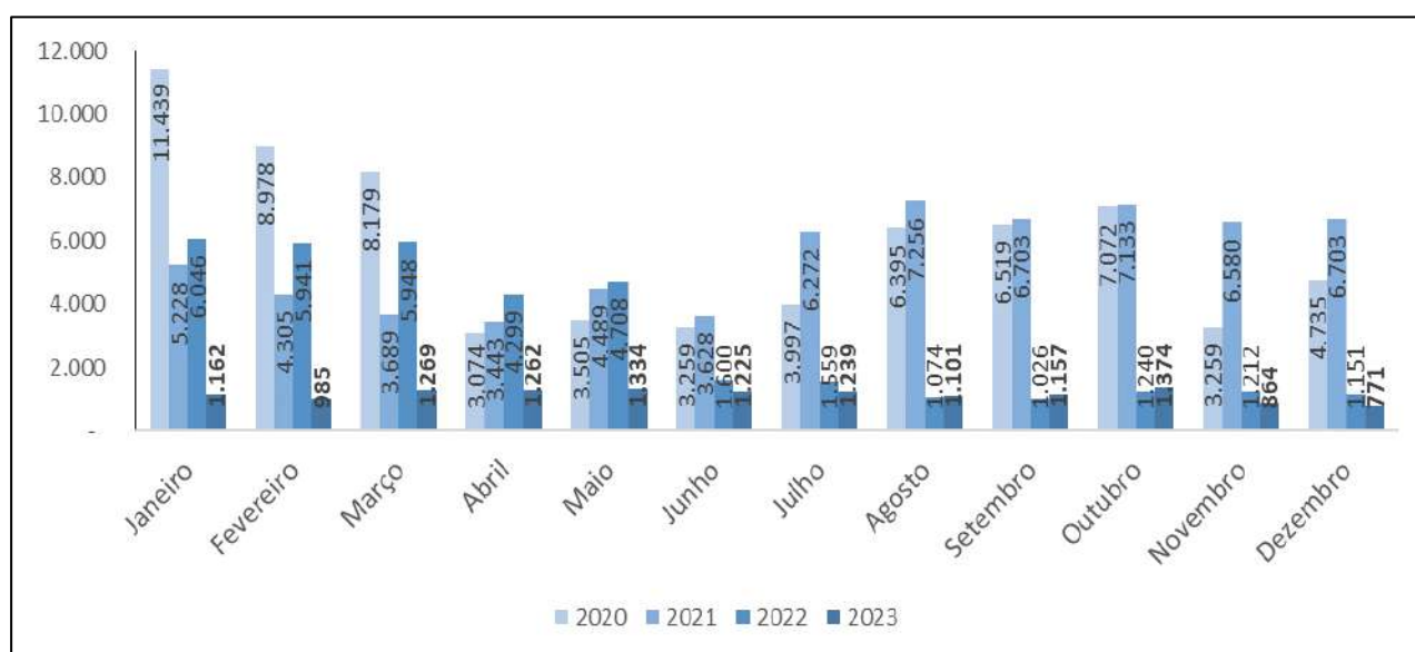
Figura 3 - Gráfico comparativo do consumo em Kwh nos anos de 2020, 2021 e 2022.
